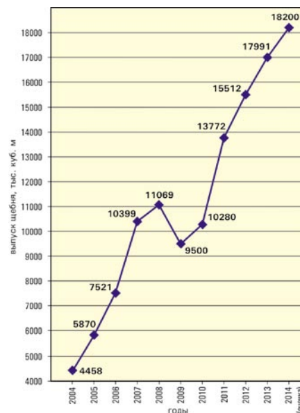
Динамика производства щебня в Республике Карелия в 2004-2014 гг.
