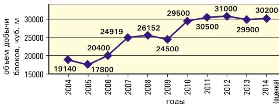
Динамика добычи каменных блоков в Республике Карелия за 2004-2014 гг.
